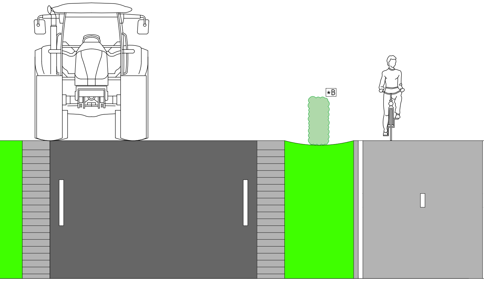
Principe profiel, Normaal Schaal: 1:50
