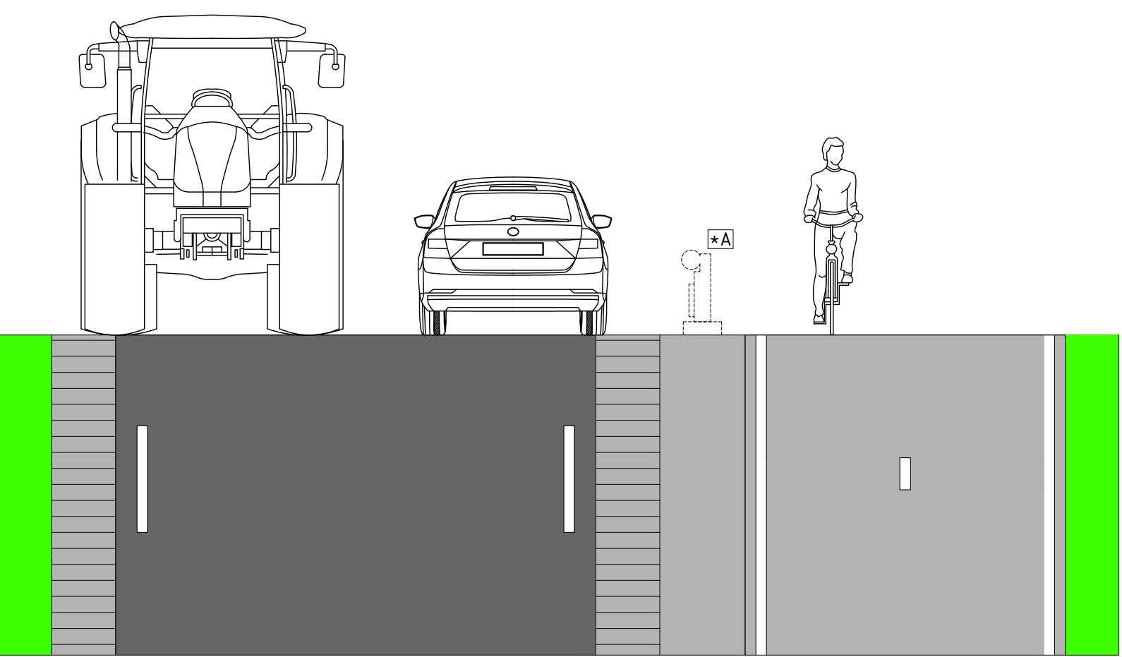
Principe profiel, Minimaal Schaal: 1:50
