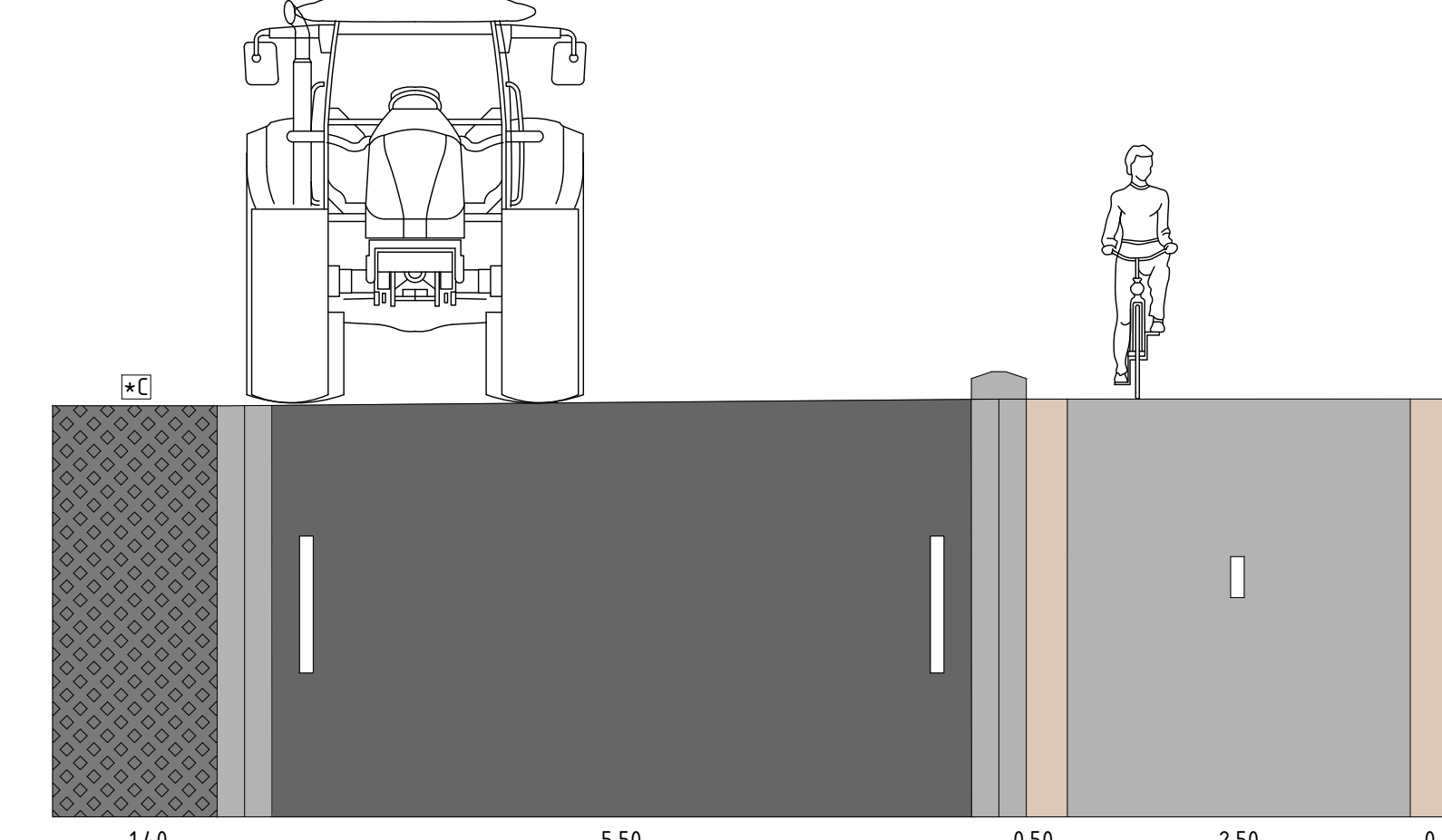
Principe profiel, Binnen de bebouwde kom Dolder Schaal: 1:50
