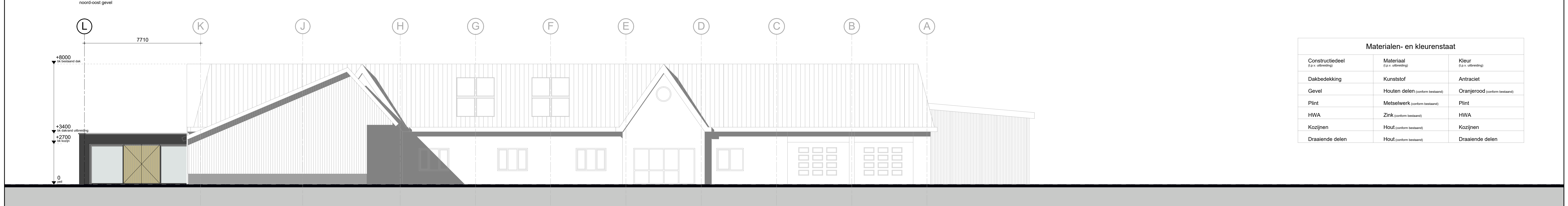
achtergevel noord-west gevel
