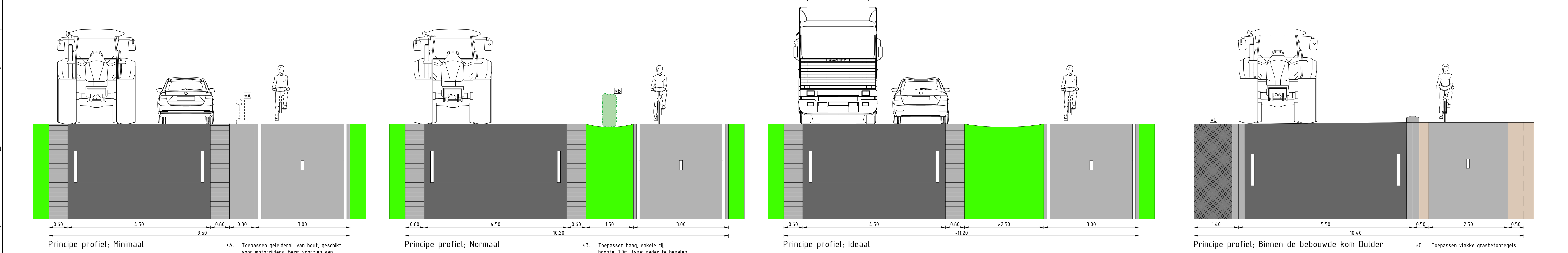
Principe profiel; Minimaal Schaal: 150 Principe profiel; Normaal Schaal: 150 Principe profiel; Ideaal Schaal: 150 Principe profiel; Binnen de bebouwde kom Dulder Schaal: 150
