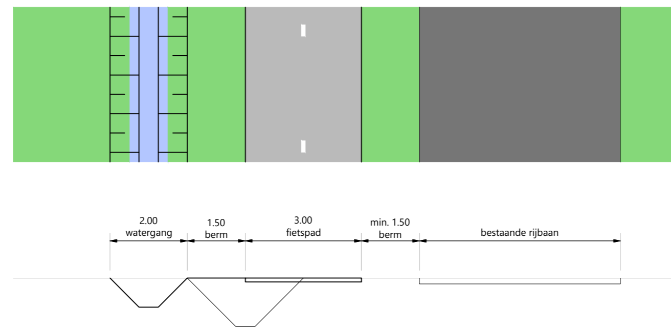
Principe profiel fietspad, berm en watergang Schaal 1:100
